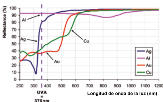
Reflectancia en% de luz reflejada para 4 metales
